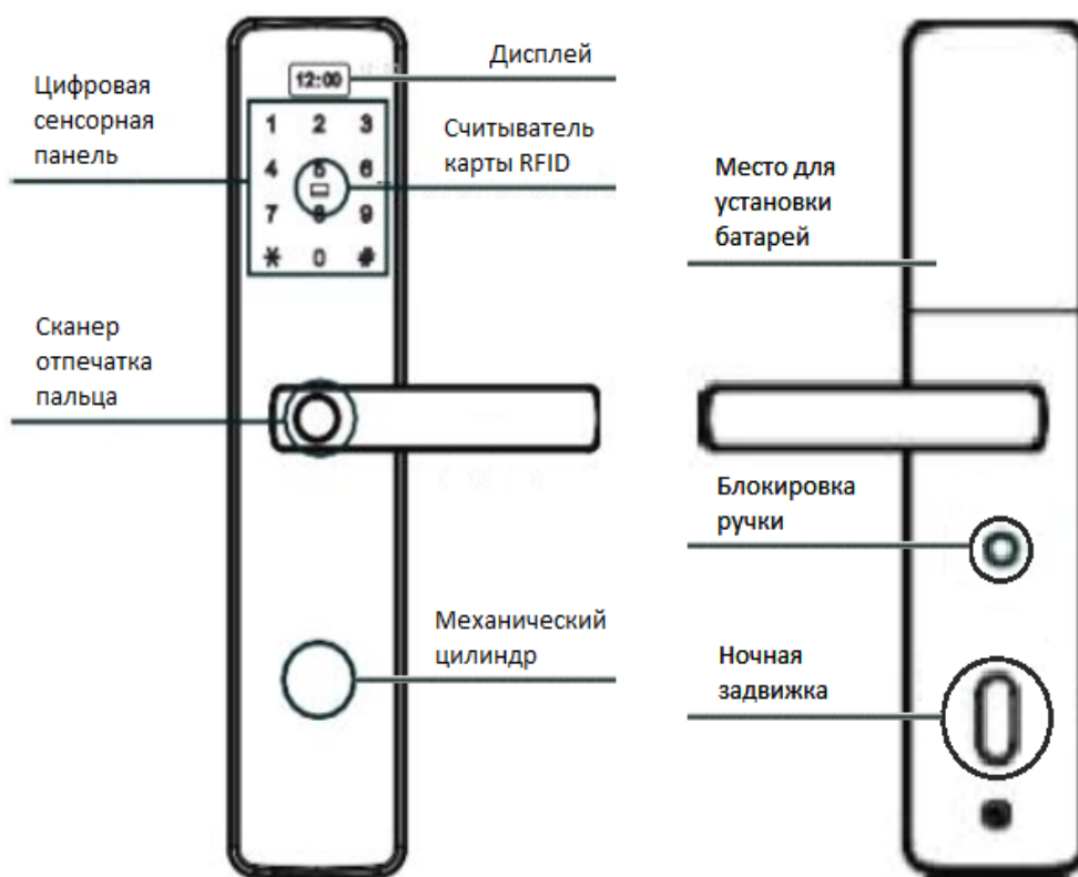
Рис. 1. Полуавтоматический замок. Устройство.
